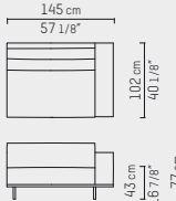
Arm right 145 cm PBC 06.103.01.--
