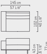
Arm left 145 cm PBC 06.103.01.--
