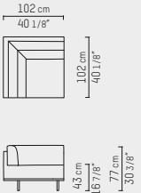
Corner 102 cm PBC 06.116.01.--
