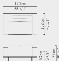
Loveseat 170 cm PBC 06.114.01.--
