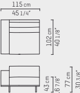
Arm left 115 cm PBC 06.102.01.--
