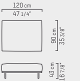
Pouf 120 x 90 cm PBC 06.110.01.--
